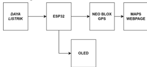
Gambar 5. Perancangan Secara Blok Diagram
