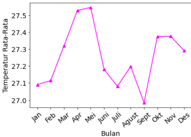
Gambar 11. Tren bulanan temperatur rata-rata
