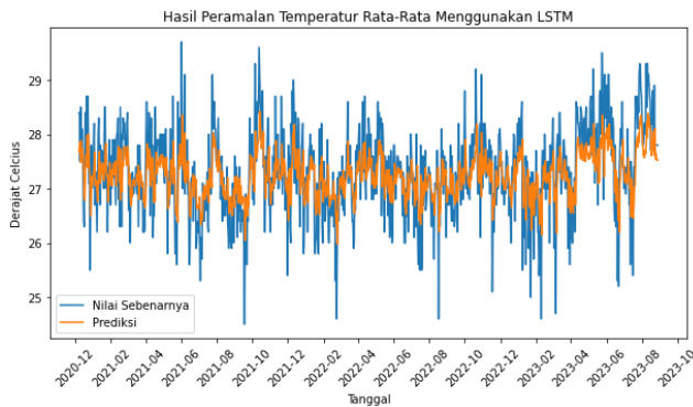
Gambar 14. Visualisasi hasil prediksi nilai temperatur rata-rata
