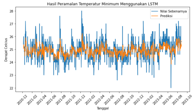
Gambar 12. Visualisasi hasil prediksi nilai temperatur minimum
