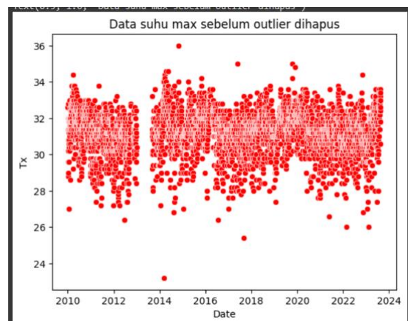
Gambar 4. Visualisasi data sebelum outlier dihapus
