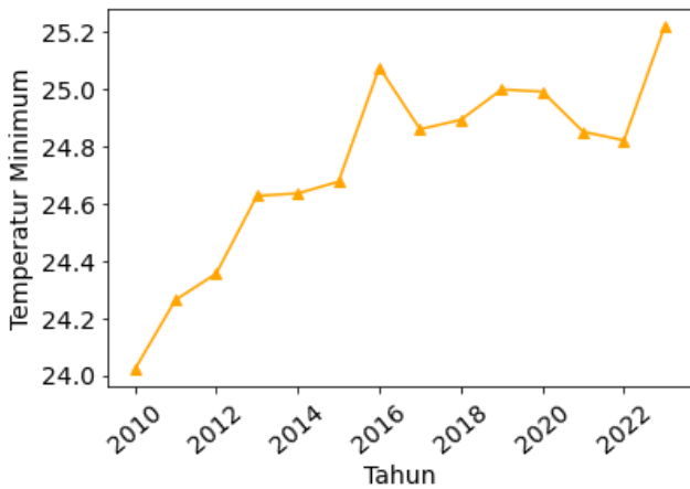
Gambar 6. Tren tahunan Temperatur minimum
