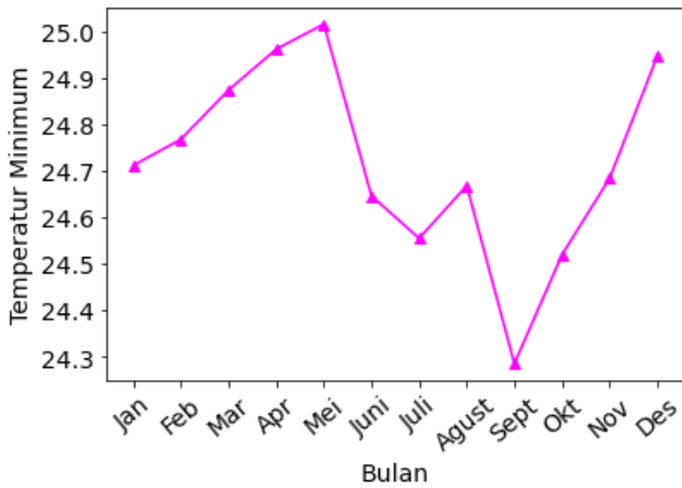
Gambar 9. Tren bulanan temperatur minimum
