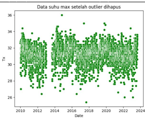
Gambar 5. Visualisasi data setelah outlier dihapus
