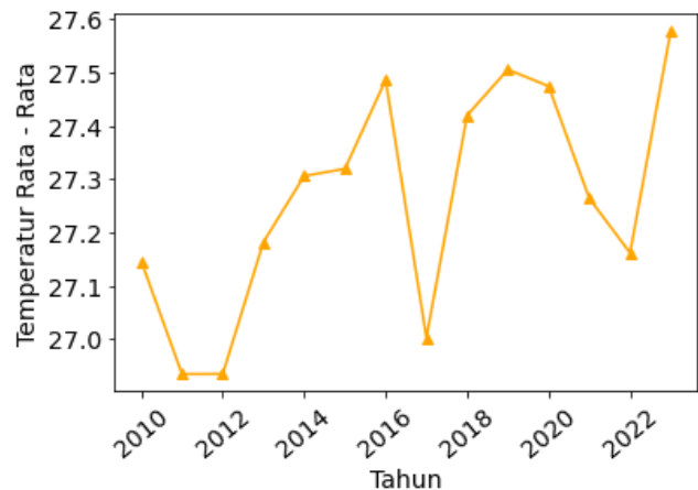
Gambar 8. Tren tahunan temperatur rata-rata
