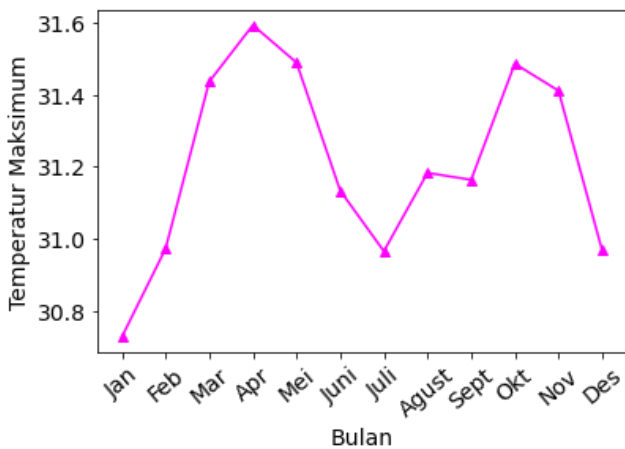
Gambar 10. Tren bulanan temperatur maksimum
