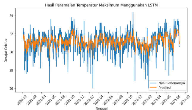
Gambar 13. Visualisasi hasil prediksi nilai temperatur maximum
