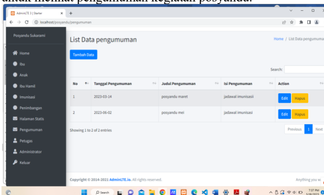
Gambar 9. Halaman Pengumuman
