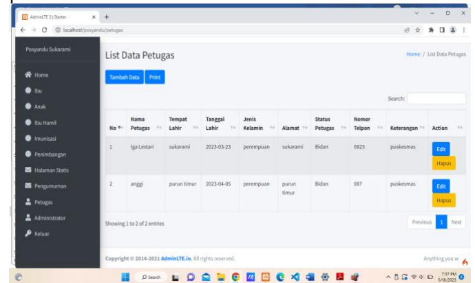
Gambar 10. Halaman Petugas
