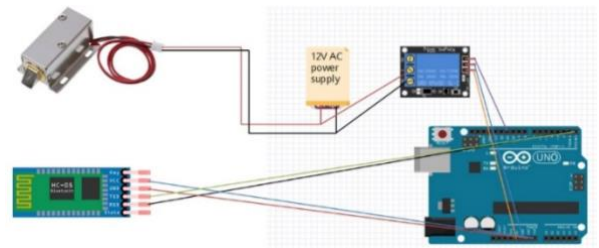
Gambar 2. Rancangan Skematik
