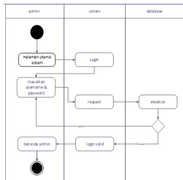
Gambar 2. Aktiviti diagram Login
