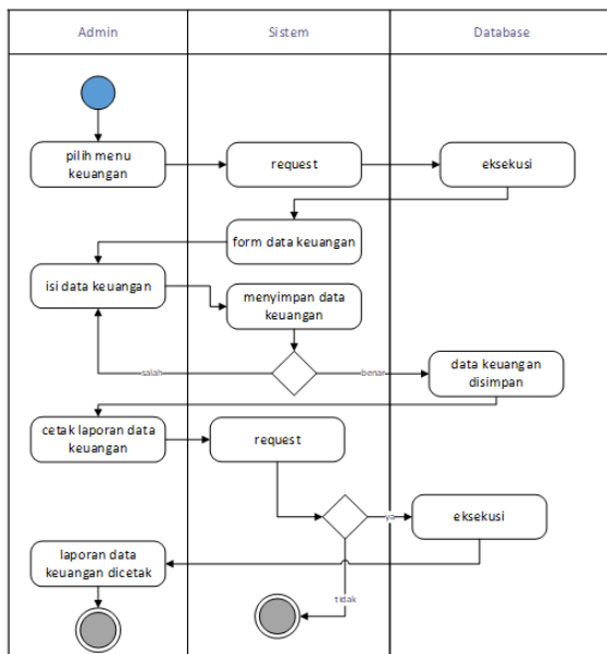
Gambar 7. Activity diagram Aktifitas surat keluar
