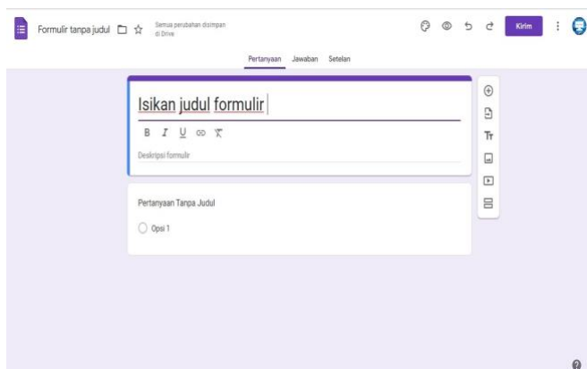
Gambar 3. Perancangan Tahap 2
