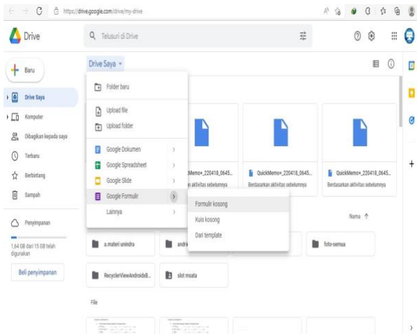
Gambar 2. Perancangan Tahap 1
