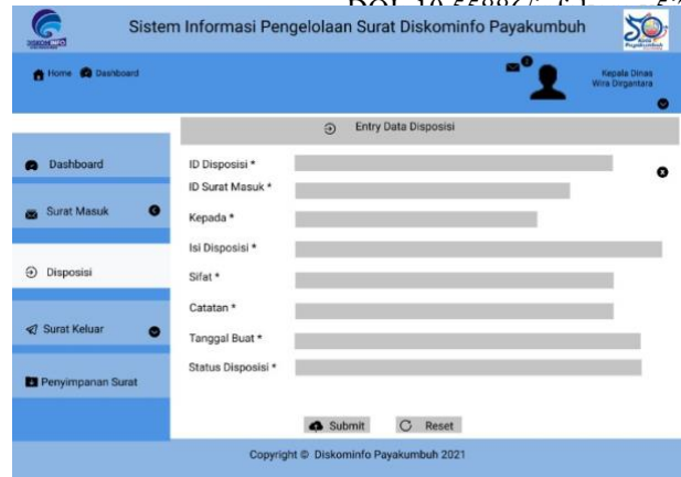
Gambar 12. Desain Interface Menu Disposisi
