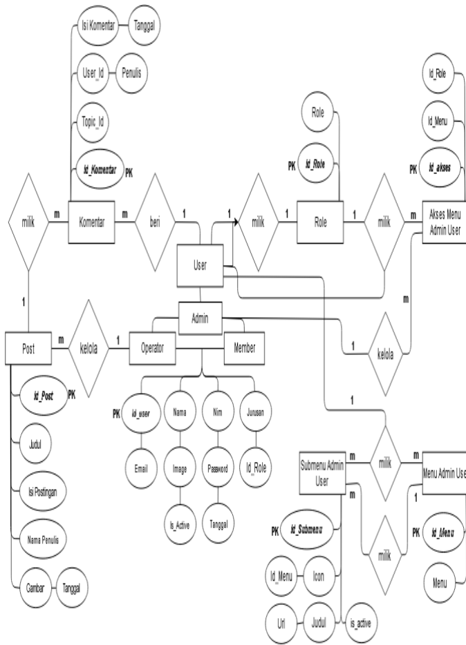
Gambar 4. ERD Sistem
